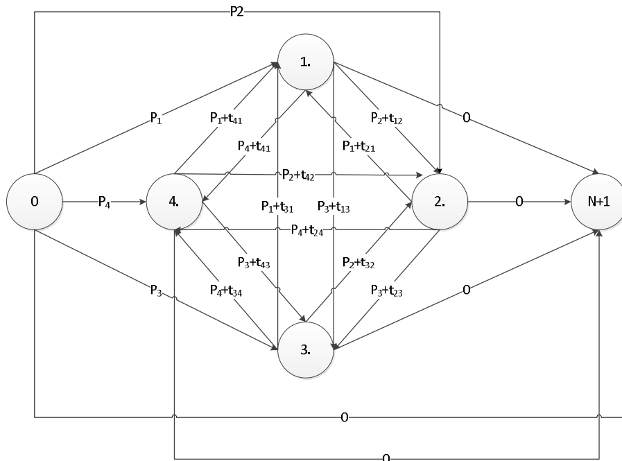
2. ábra: A probléma vázolására alkalmazott gráf
