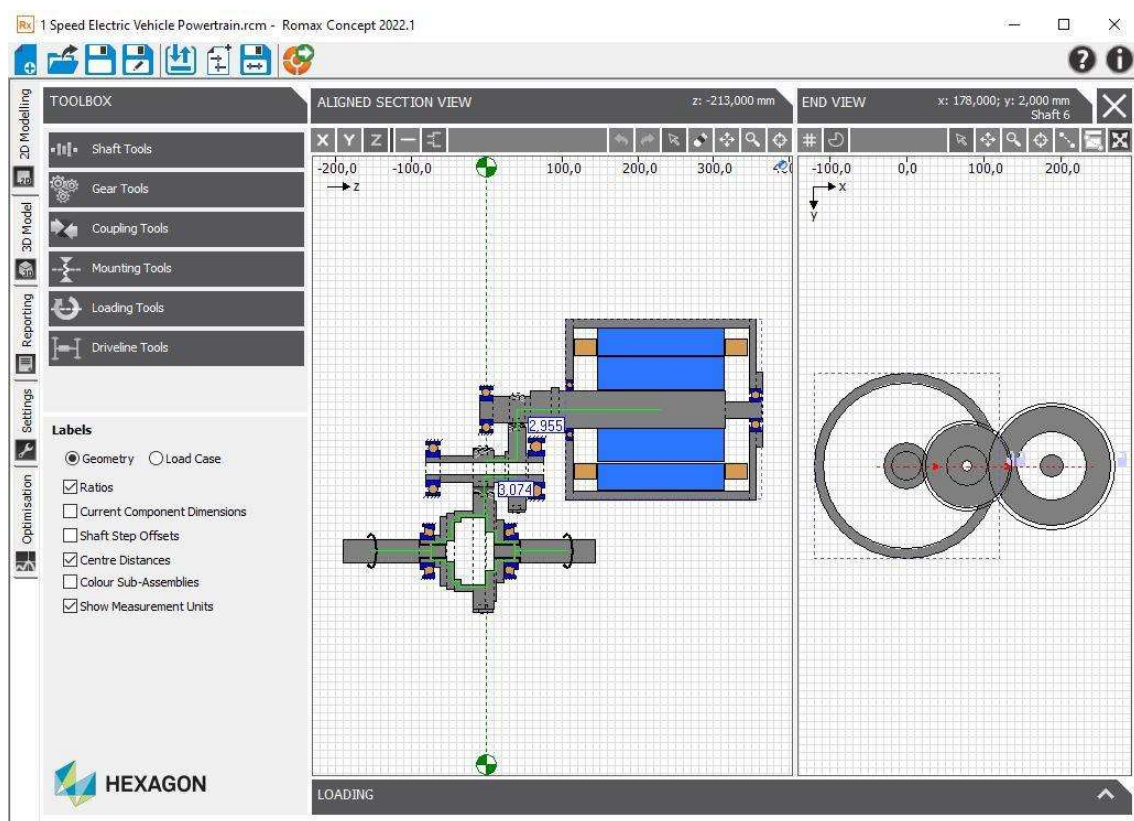
1. ábra: egy elektromos járműhajtás 2D modellje a Romax Concept szoftverben
