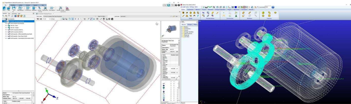
2. ábra: Elektromos járműhajtás modellje, balra Romax, jobbra Adams
