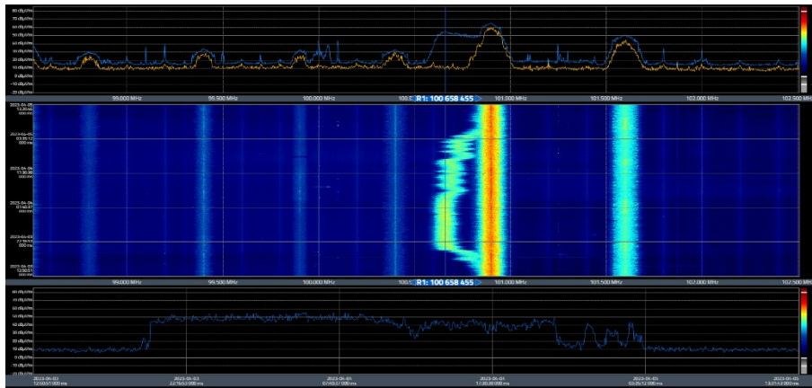
4. ábra Rádióadó meghibásodása miatt keletkezett zaj.
