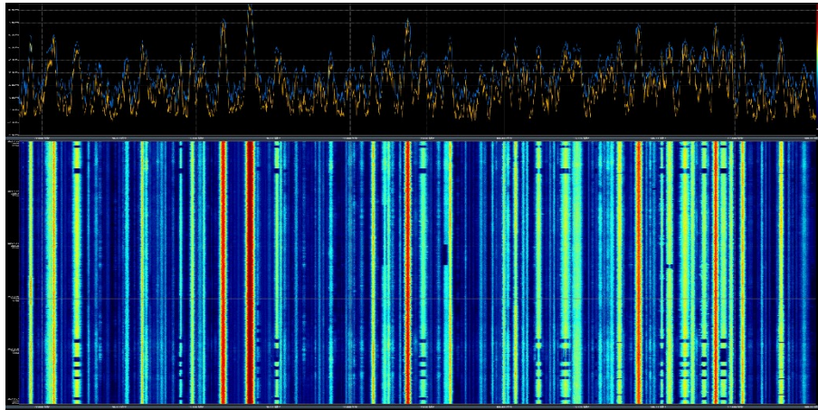
1. ábra 87,5 MHz - 108 MHz közötti frekvenciasáv (FM sáv) spektrogramja. Az x tengely a frekvencia, y tengely az idő és a szín reprezentálja a vételi térerősség értékét. Az egyes függőleges vonalak egy-egy rádióadást mutatnak. A diagram feletti grafikon ábrázolja a térerősség maximumokat és a vételi térerősség átlagát.
