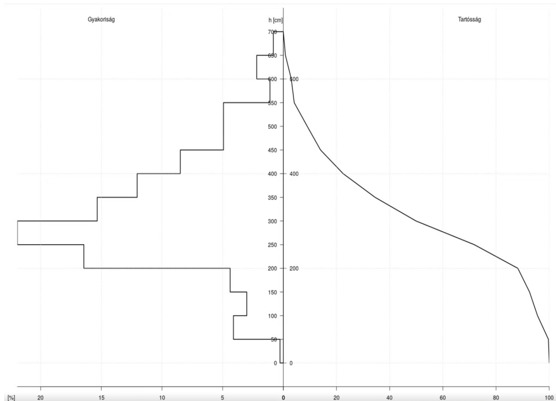
9. ábra: Gyakoriság-tartósság grafikon
