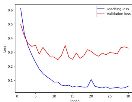
5. ábra Háromrétegű neurális háló tanulási és veszteség függvénye az a) és tanulási és validációs pontossága a b) ábrán láthatók (Takács S. L., 2023).
