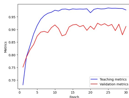
5. ábra Háromrétegű neurális háló tanulási és veszteség függvénye az a) és tanulási és validációs pontossága a b) ábrán láthatók (Takács S. L., 2023).
