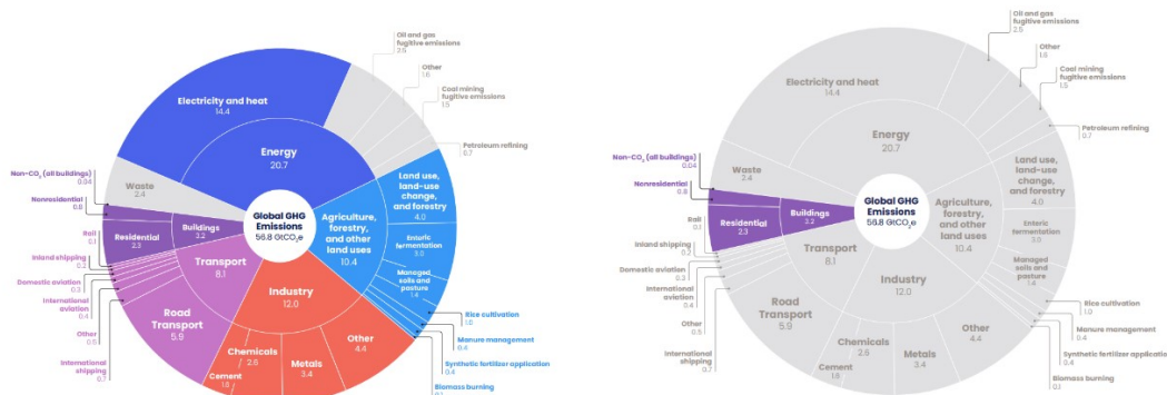
1. diagram Globális nettó antropogén ÜHG-kibocsátás ágazonként 2021-ben [1]
