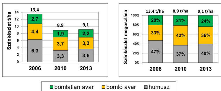
4. ábra: Három év lombhullás után gyűjtött mintáinak átlagos szénkészlete és annak megoszlása (Forrás: saját mérési adatok alapján)
