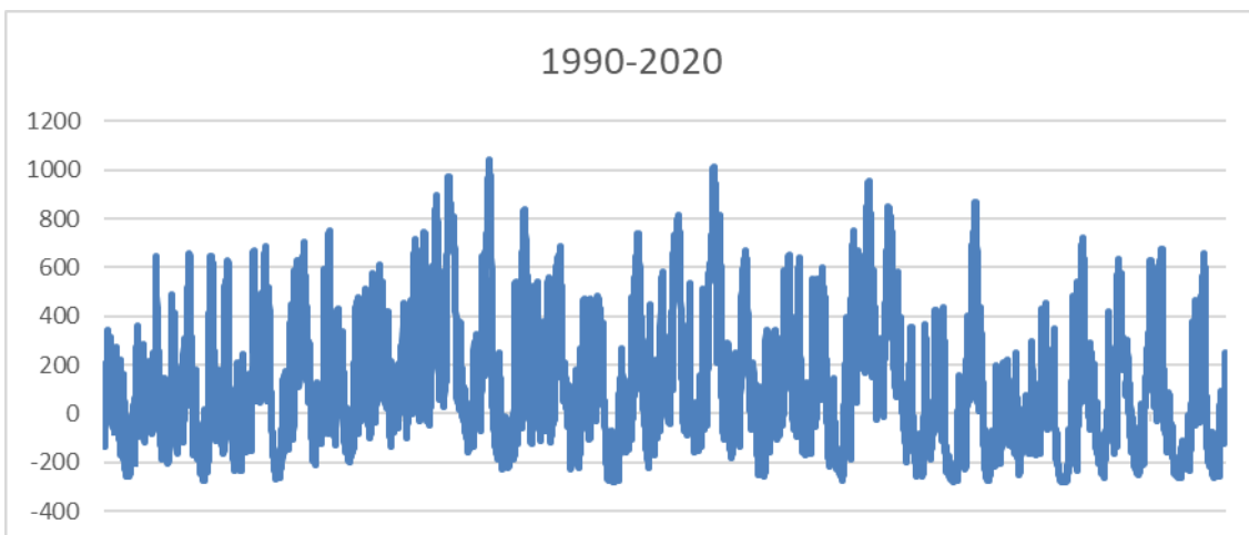
8. ábra: A Tisza 100 éves hidrológiai időszora 30 éves lebontásokban (saját diagramm a szolnoki KÖTIVIZIG rendelkezésre bocsátott adataiból) A vízszintes tengely a jelölt időszakot (év), a függőleges tengely a mért adatot (cm) jelöli.
