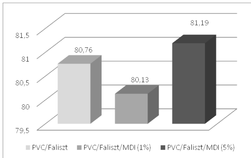
1. ábra: Az eltérő kompozitok keménységi értékeinek változása
