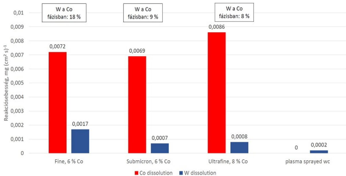
3.2.3. ábra. Co és W oldódási sebességének összehasonlítása keményfémeken és plazmaszórással készült, Co mentes WC mintán
