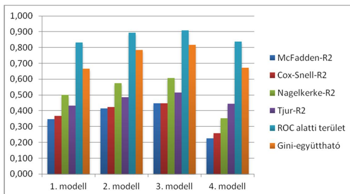
1. ábra: Az egymásba ágyazott modellek illeszkedési mutatói
